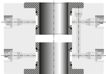
Boccola hydro con ingrassatori RADIALI RADIAL alignment of grease nipples RADIALE Anordnung der Schmiernippel
